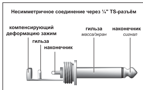
Рис. 6.2: 6,3-мм моноштекер
