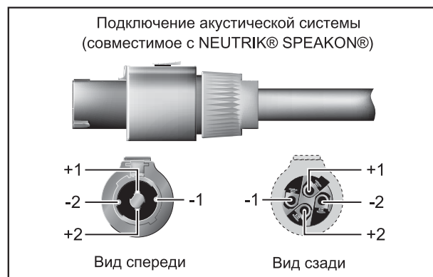
Рис. 6.1: Штекер Speakon®
